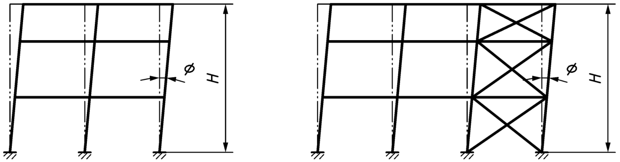
Рисунок 7.4 – Початкова недосконалість, що спричиняє розхитування
