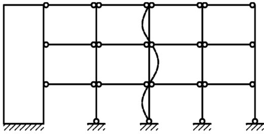
(a) Форма втрати стійкості елемента без розхитування
