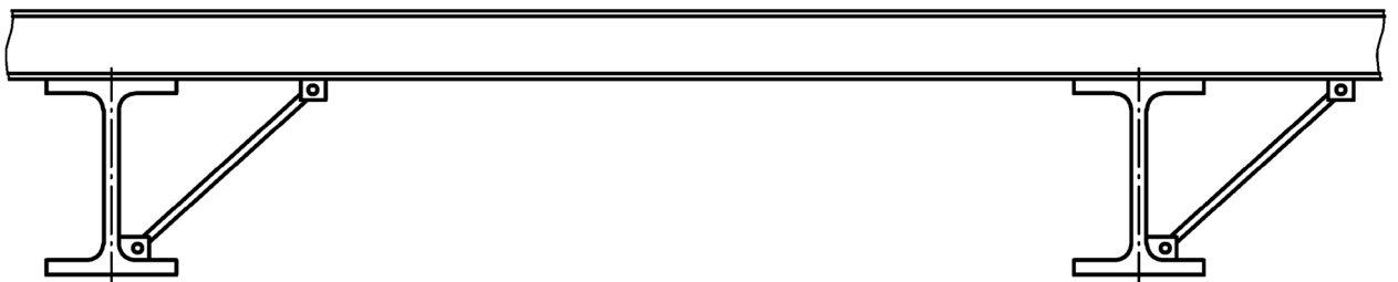
Рисунок 8.8 – Типове жорстке закріплення від кручення
