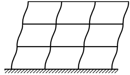
(b) Форма загальної втрати стійкості з розхитуванням
