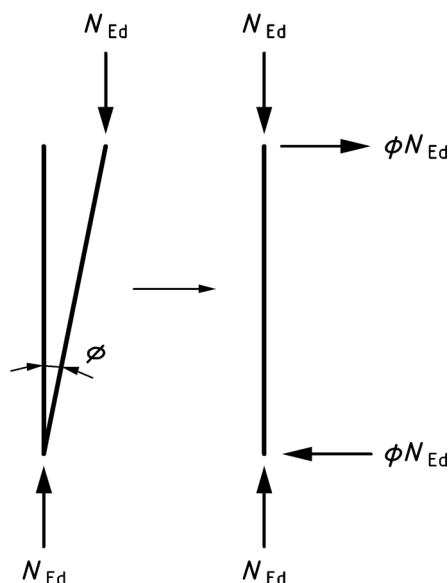
Рисунок 7.5 – Заміна початкової недосконалість, що спричиняє розхитування, на еквівалентні горизонтальні сили
