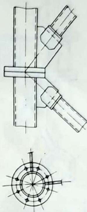
10. Узел примыкания распорок и раскосов к поясам башни РРЛ
