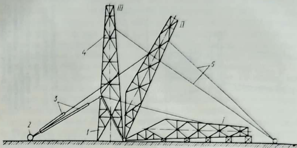
Рис. 56. Монтаж башни способом поворота:
