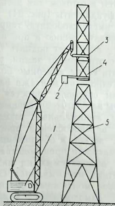
Рис. 32. Монтаж башни способом наращивания:
