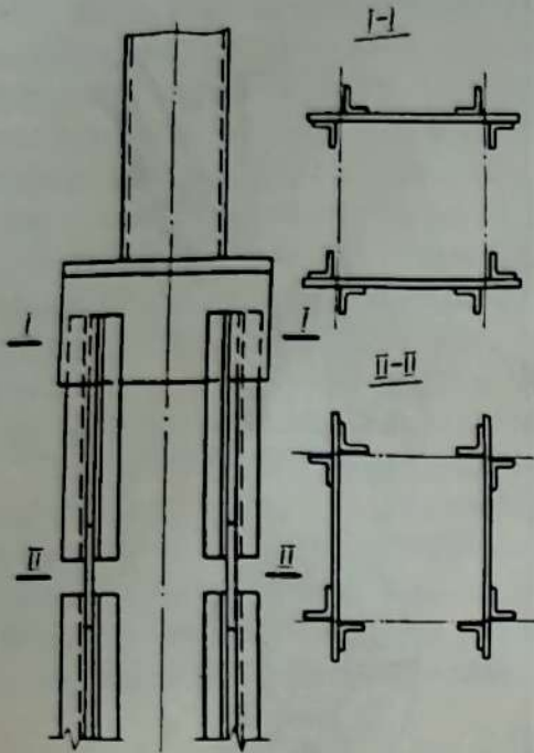
5. Опорный узел с переходными деталями из уголков *
