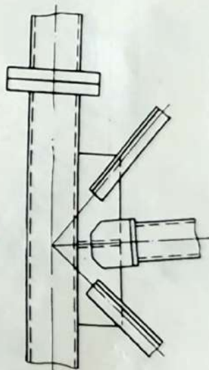
12. Узел примыкания распорок и раскосов к поясам башни (с вынесенным стыком)
