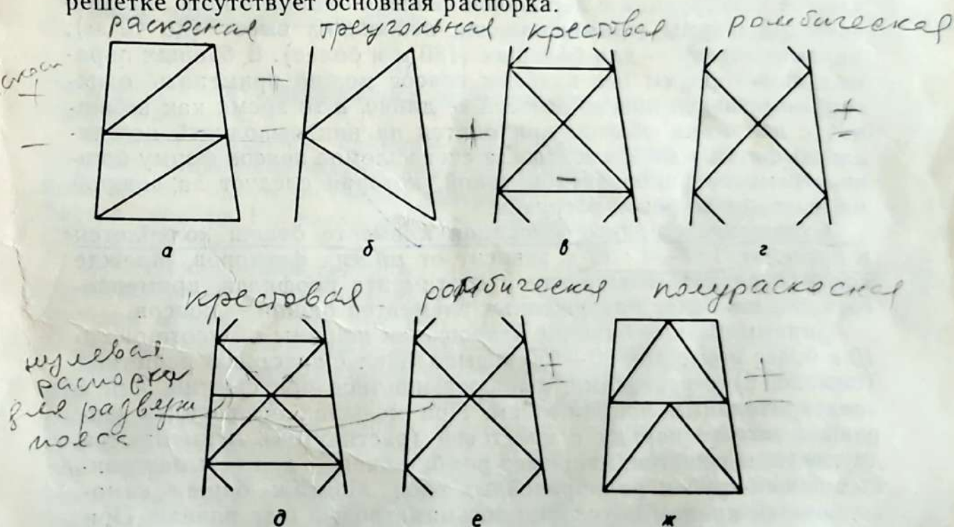
Рис. 5. Типы решеток стальных башен:
