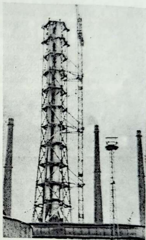
Рис. 54. Смонтированная часть башни-трубы прислонным краном БК-300П.
