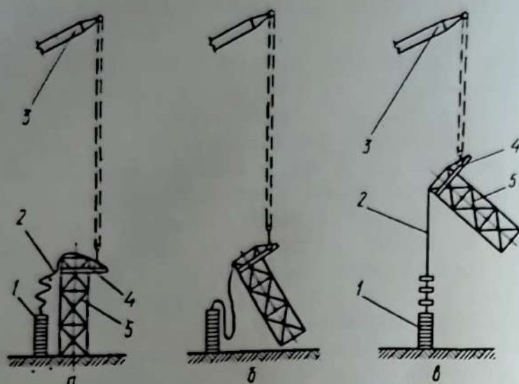
Рис. 55. Монтаж верхних блоков
