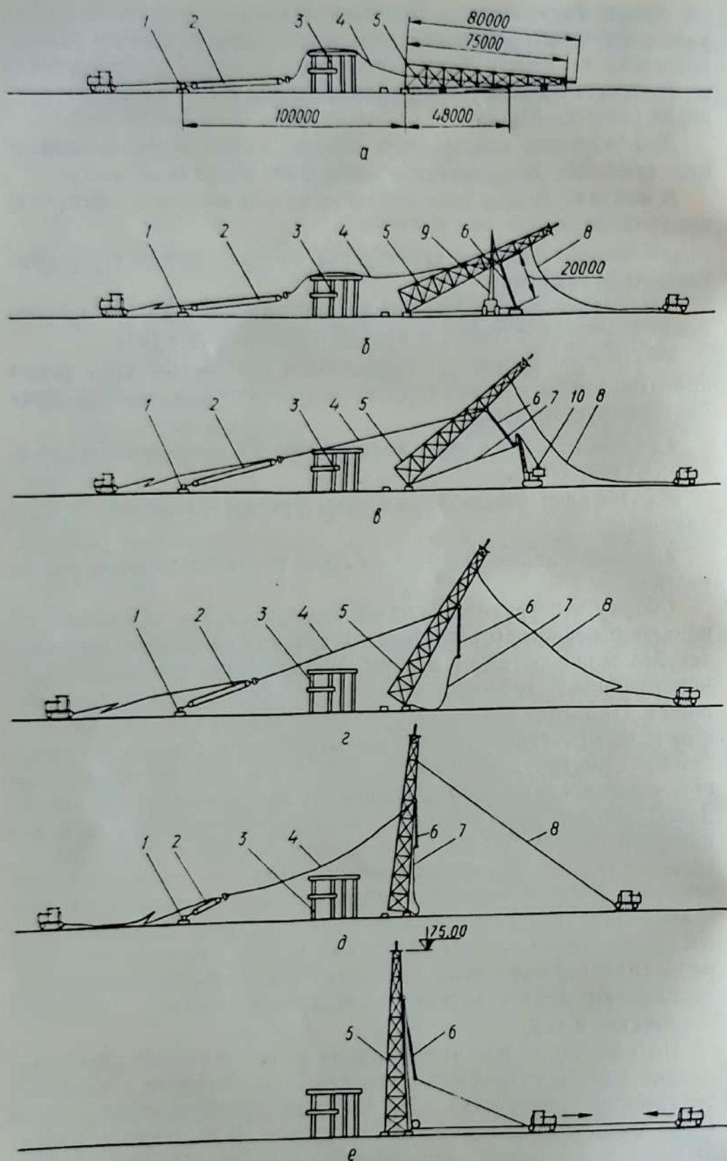
Рис. 39. Этапы монтажа башни (а—е):
