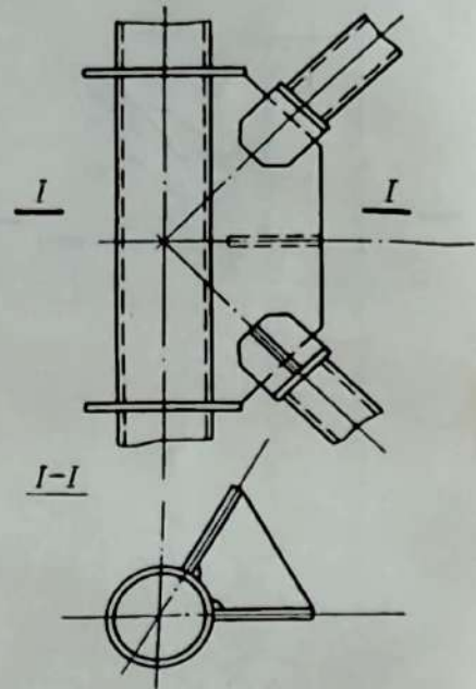
14. Узел примыкания распорок и раскосов к поясам башни с окаймлением фасонок
