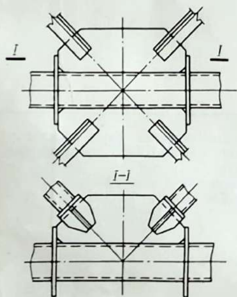
19. Узел пересечения раскосов с промежуточными распорками с раскосами из уголков
