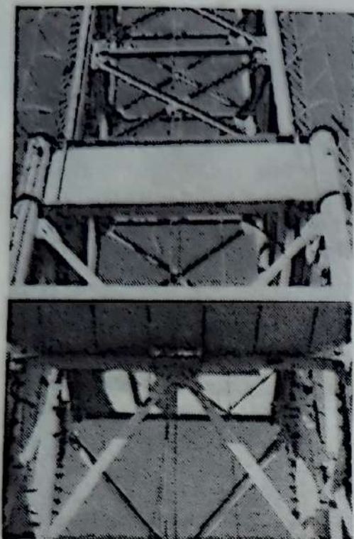
Рис. 76. Ярус с замкнутым контуром двутавровых балок.
