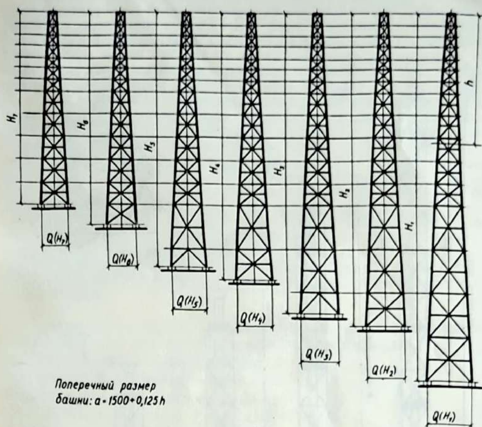
Рис. 6. Башни для антенн СГД РА (унификация типоразмеров схемы).
