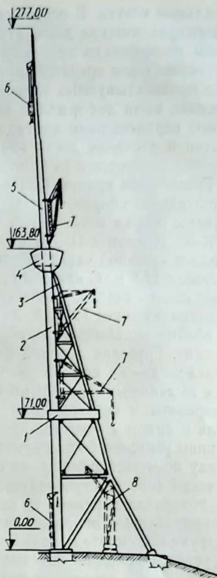
Рис. 44. Монтаж башни Тбилисского телецентра:
