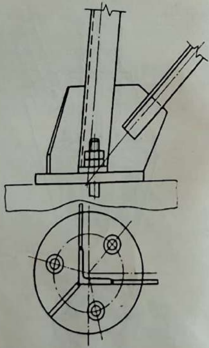
8. Опорный узел башни с поясами из одиночных уголков
