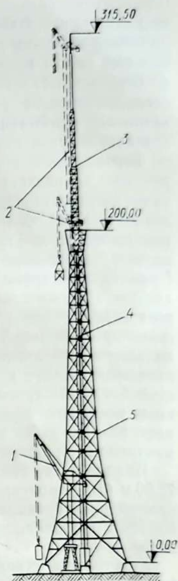
Рис. 45. Монтаж башни Ленинградского телецентра:
