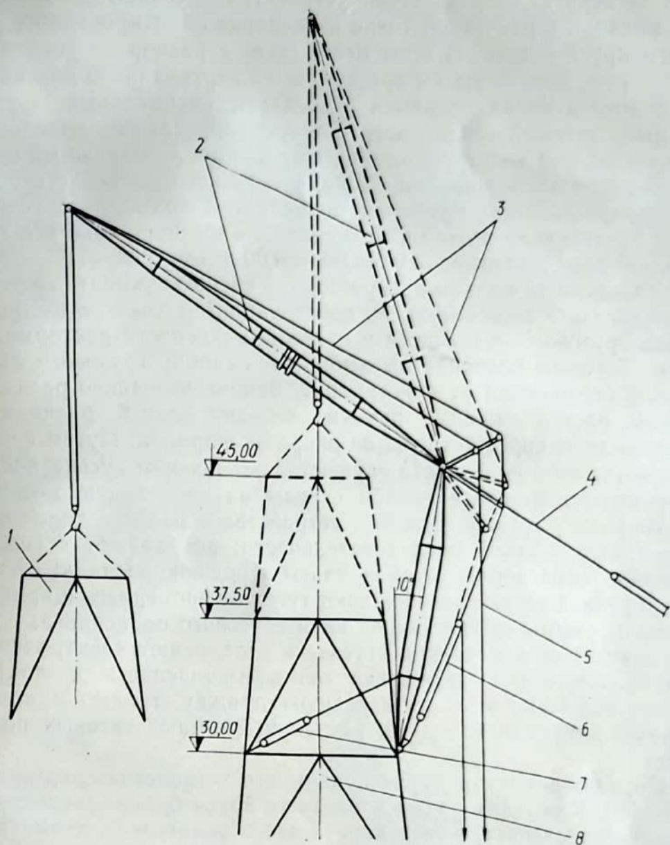
Рис. 50. Монтажное устройство с использованием БСО крана МКГ-25БР:
