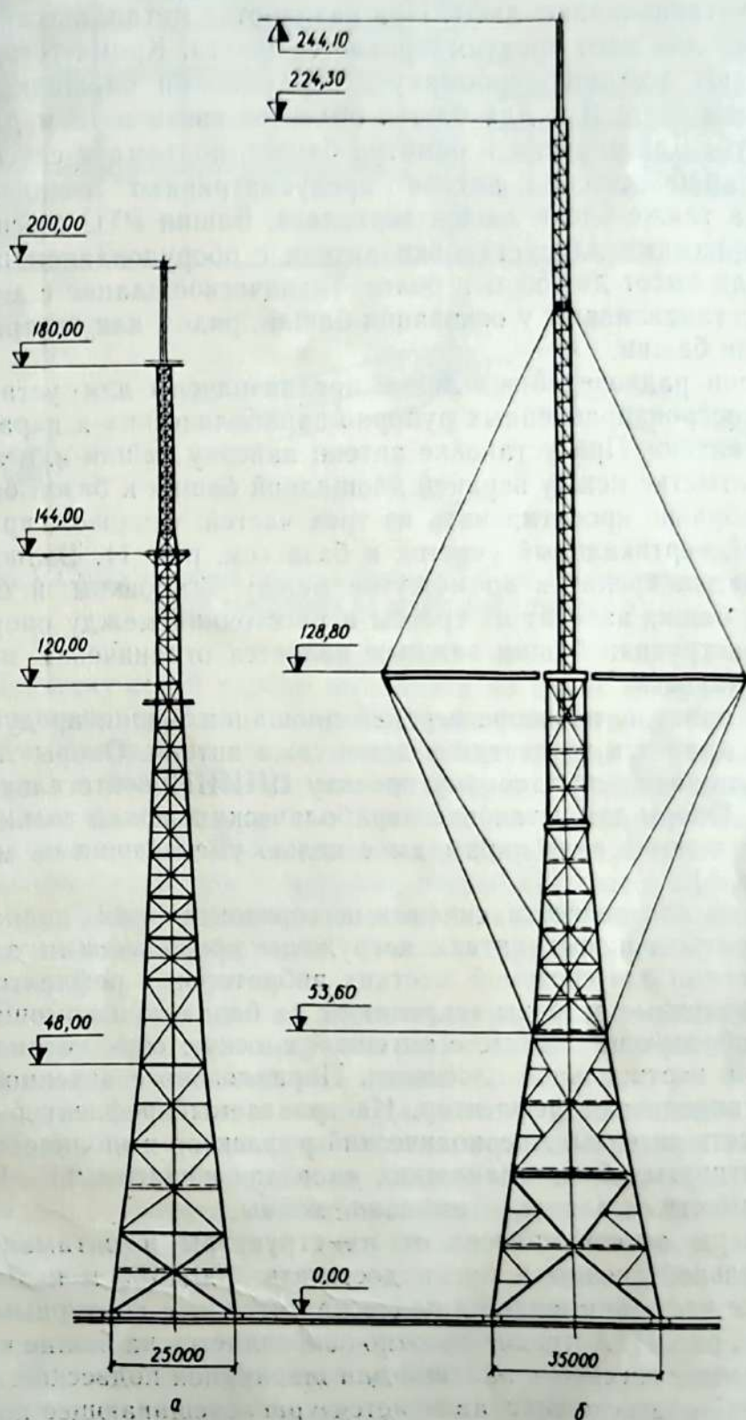
Рис. 3. Схемы башен для РТС:
