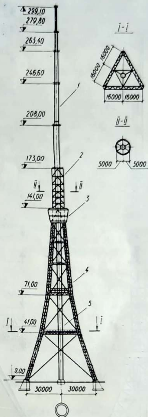
Рис. 13. Схема телевизионной башни в Ереване:
