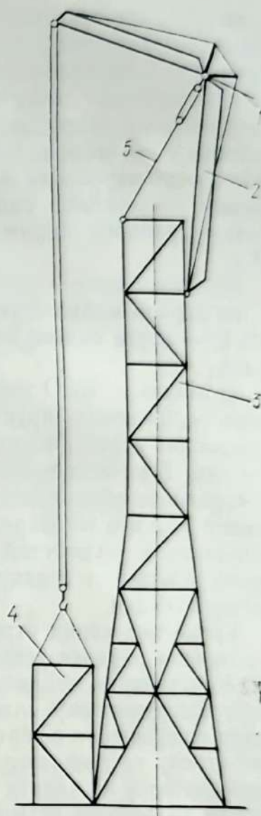
Рис. 49. Монтаж верхней части башни закрепленным башенно-стреловым оборудованием гусеничного крана:
