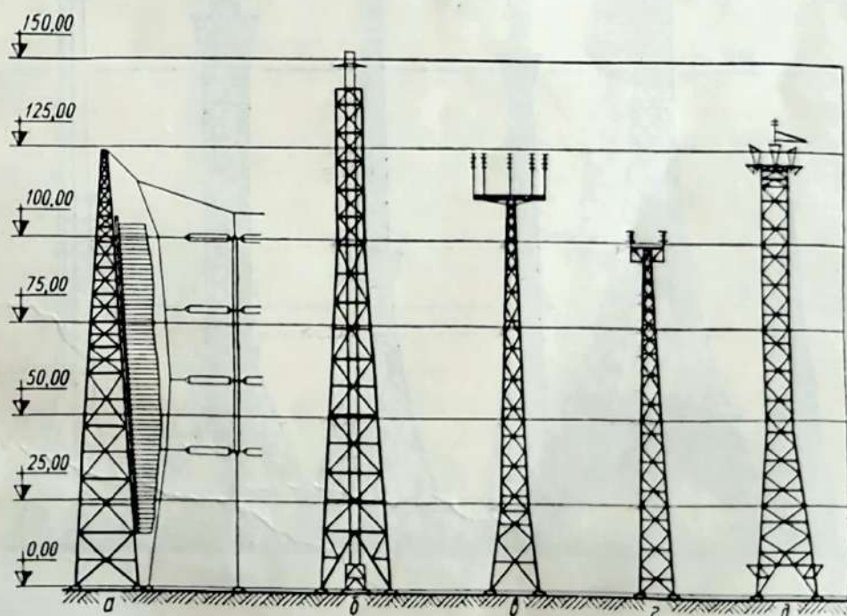
Рис. 1. Типы башен:
