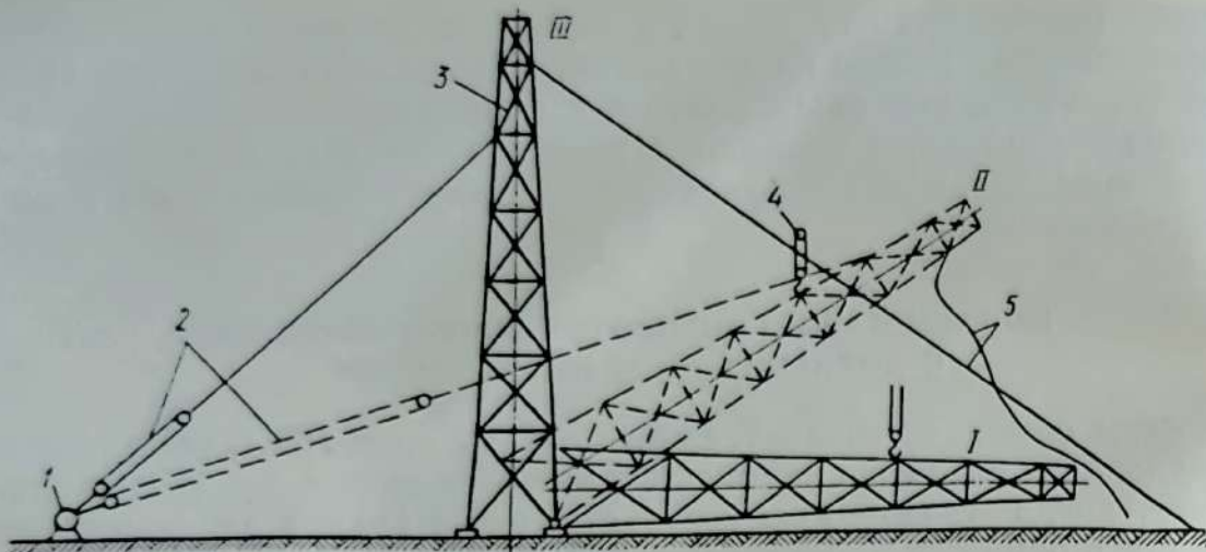
Рис. 36. Монтаж башни поворотом вокруг шарниров с дотягиванием полиспастом:
