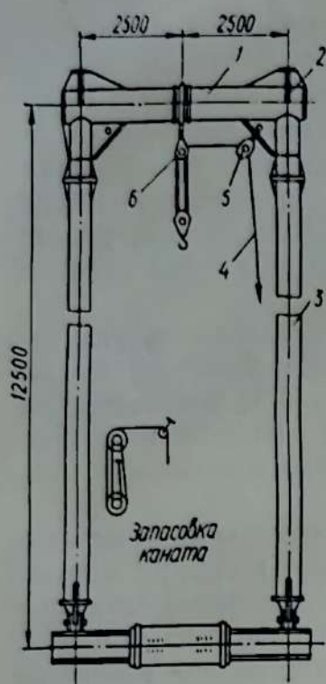
Рис. 46. Переставной портал:
