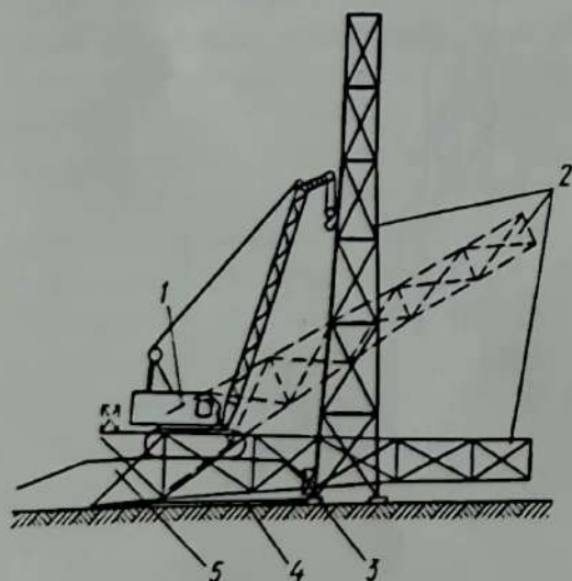
Рис. 34. Монтаж стреловым краном башни, собранной на земле:
