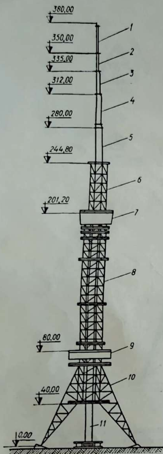
Рис. 14. Схема телевизионной башни в Киеве:
