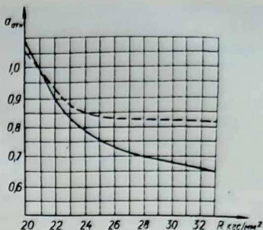
Рис. 30. Зависимость относительной величины поперечного размера башни от расчетного сопротивления стали.
