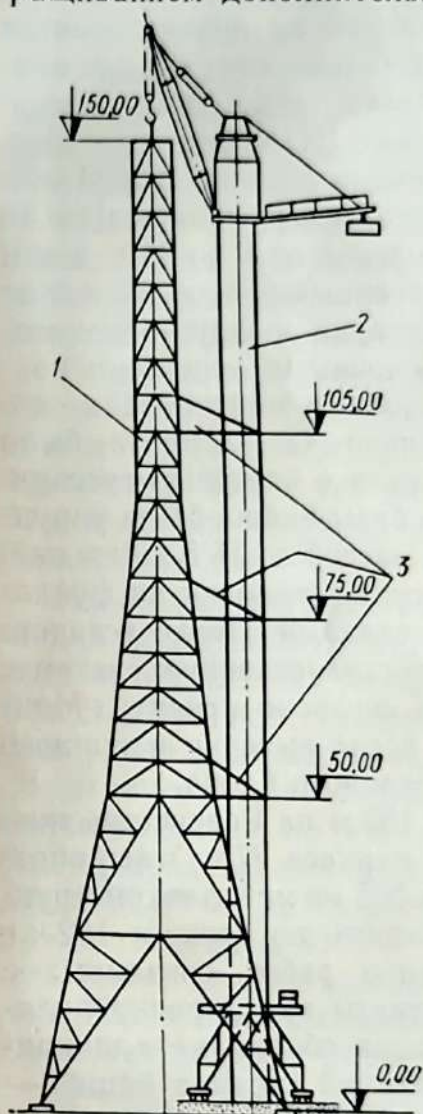
Рис. 53. Монтаж башни прислонным башенным краном: 1 — башня; 2 — кран прислонный; 3 — диафрагмы.
