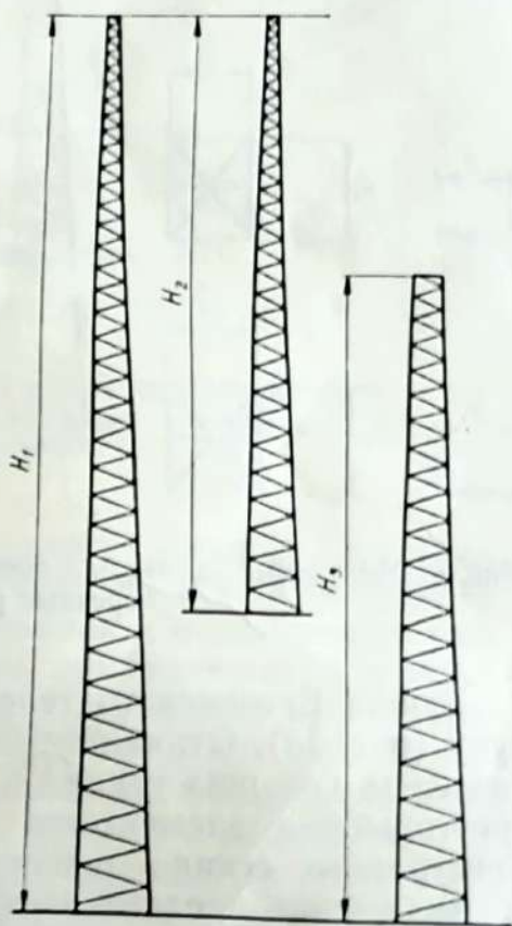
Рис. 8. Модульные схемы для построения башен различных высот.
