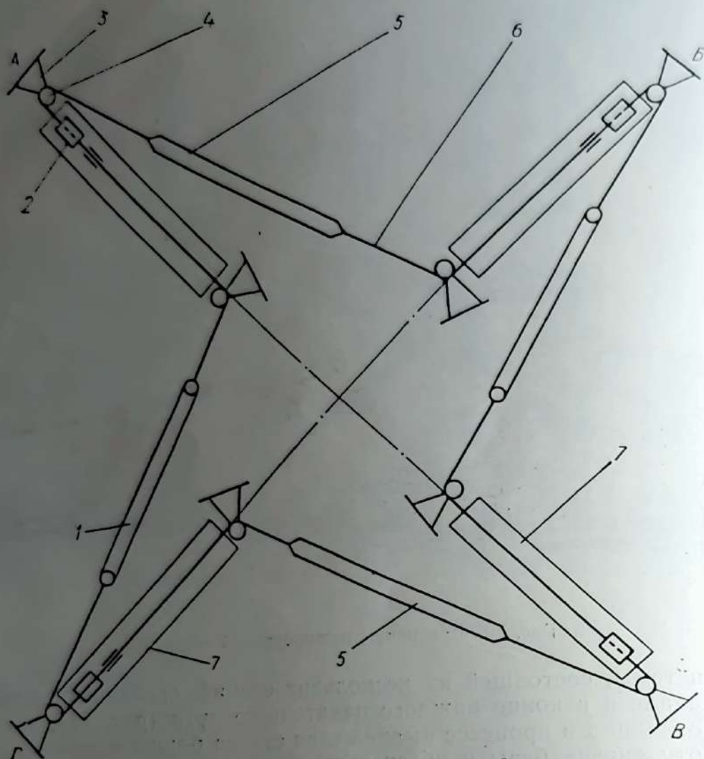
Рис. 71. Синхронизирующе-натяжное устройство:
