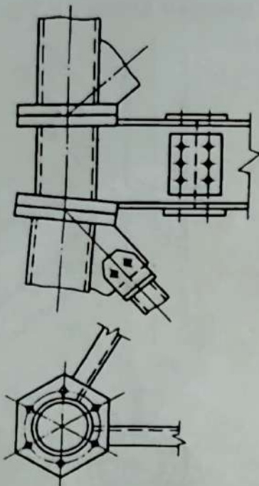
13. Узел примыкания распорок и раскосов к поясам башни РРЛ в пос. Тараща
