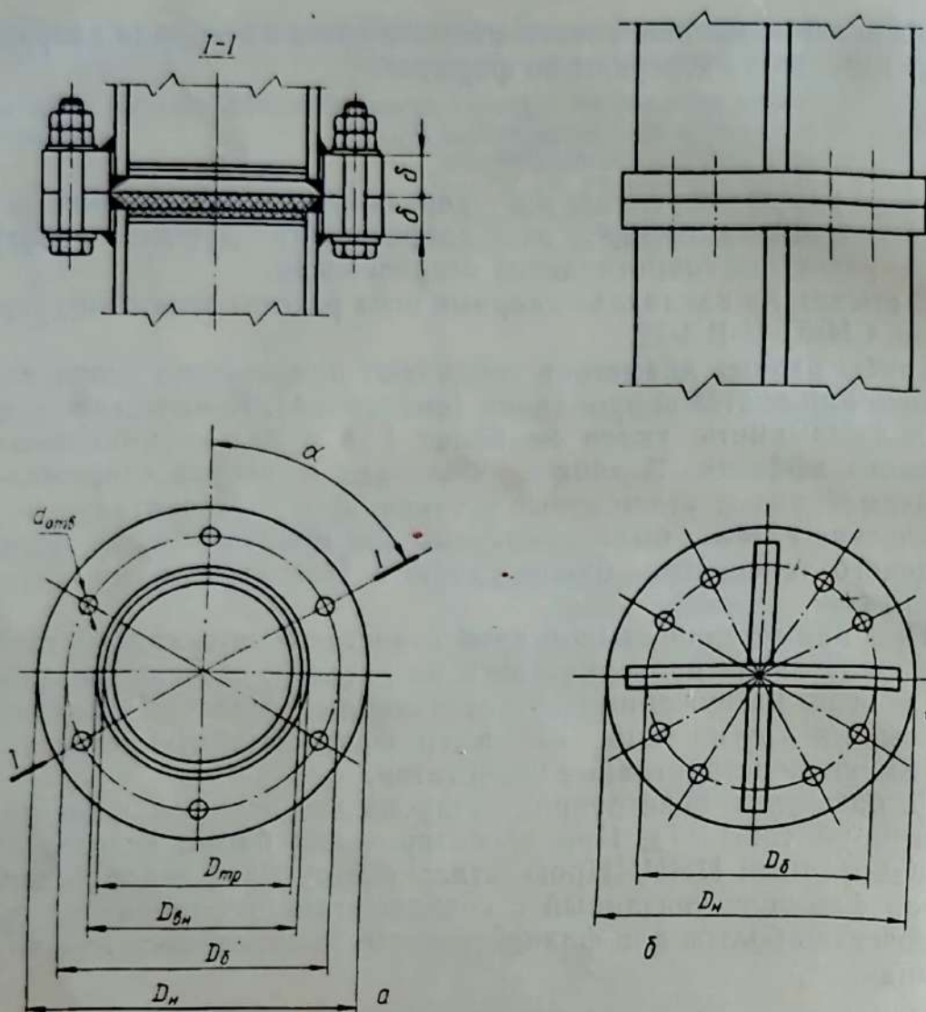
Рис. 17. Фланцевые стыки элементов башен: а — стык трубчатого элемента; б — стык элемента из сварного крестового сечения.
