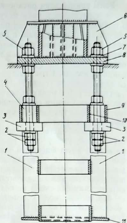
Рис. 16. Закладная деталь для крепления башмака пояса к фундаменту:
