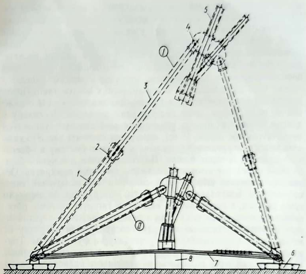
Рис. 66. Схема работы тормозного приспособления:
