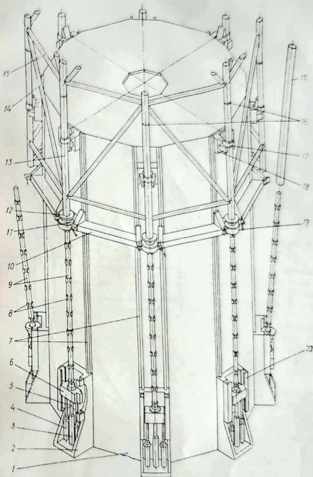
Рис. 72. Гидроподъемное устройство:
