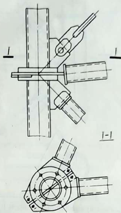
11. Узел примыкания распорок и раскосов к поясам башни-трубы для химического производства
