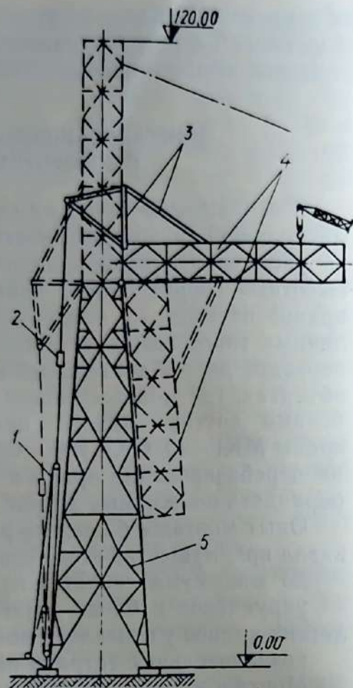
Рис. 81. Монтаж башни способом наращивания с поворотом ее верхней части:
