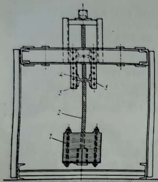
Рис. 19. Динамический гаситель колебаний:
