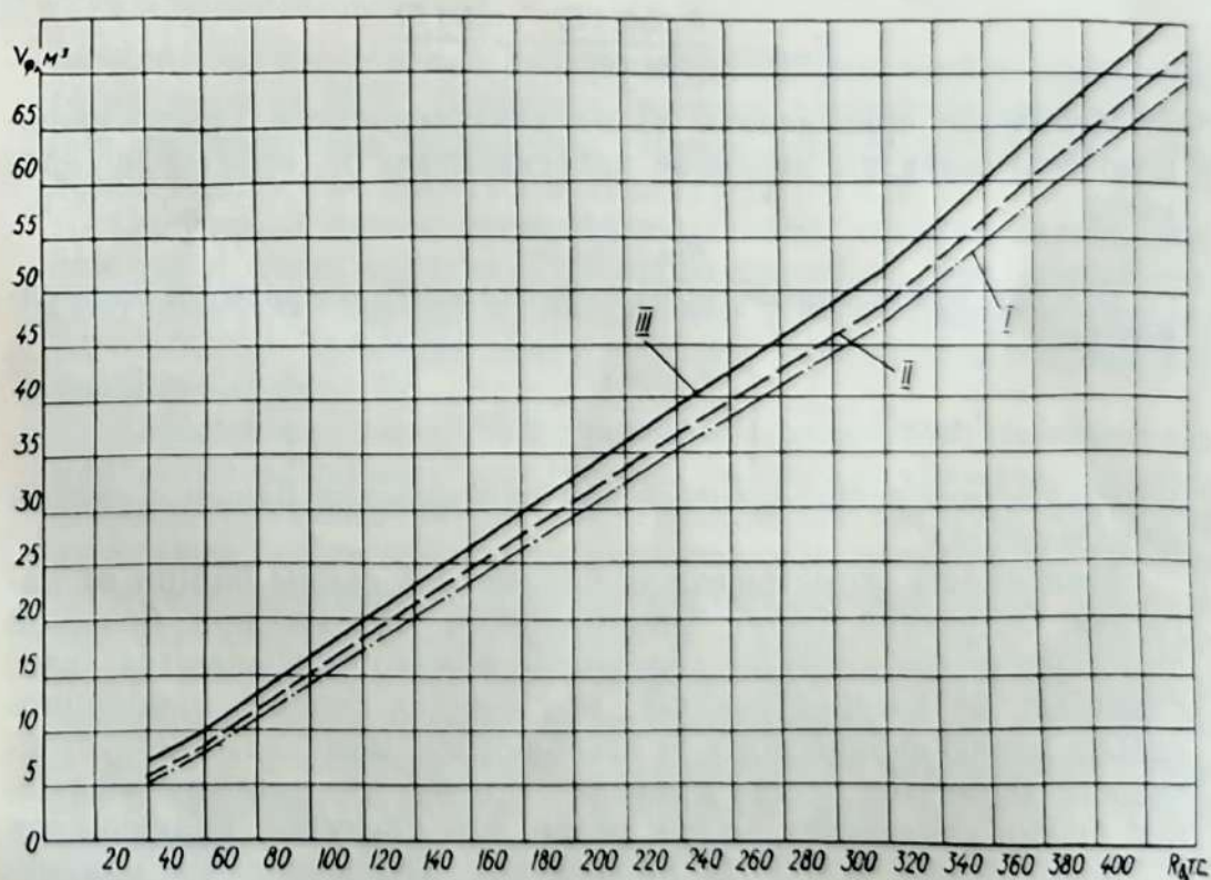
Рис. 27. Зависимость объема фундаментов V_{\text{ф}} от вырывающей силы R_{\text{в}} : I — III — типы грунтов.
