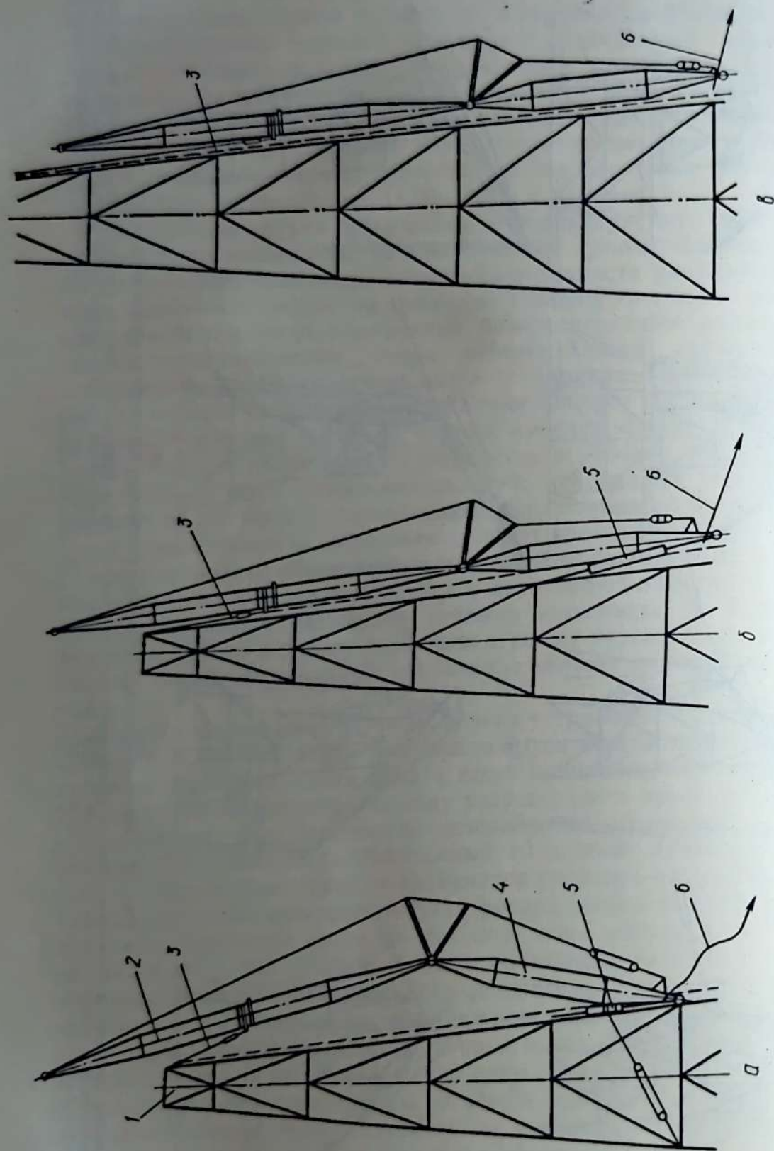
Рис. 52. Демонтаж грузоподъемного устройства:
