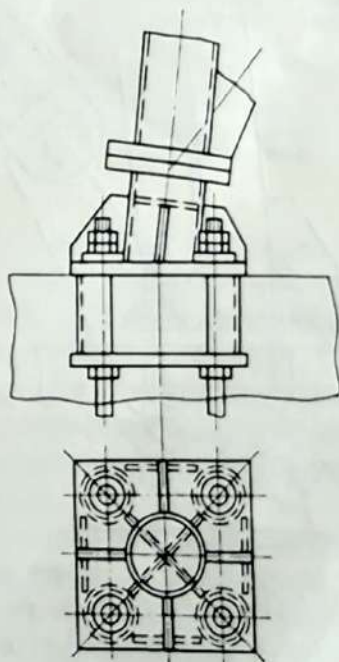
4. Опорный узел башни радиорелейной линии (с переходной деталью)
