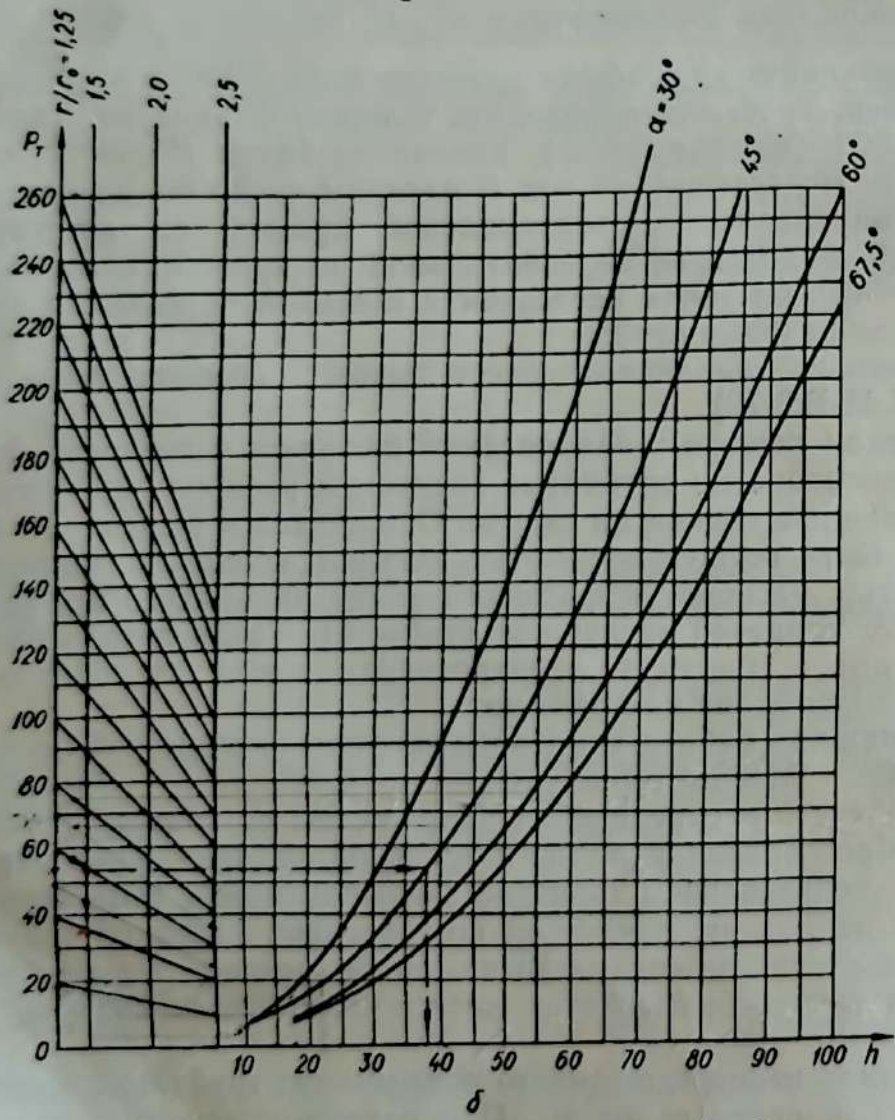
Рис. 18. Зависимость толщины плиты от усилий в болтах: а — расчетная схема разрушения плиты; б — графики зависимости усилий P_T от толщины h .
