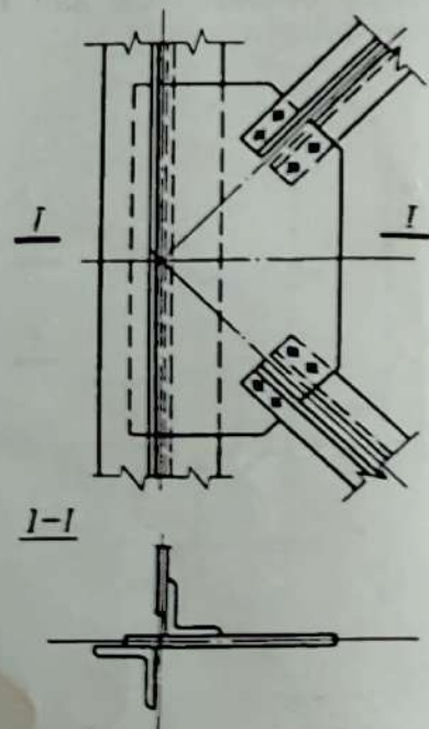
16. Узел примыкания распорок и раскосов к поясам башни (с элементами из уголков)
