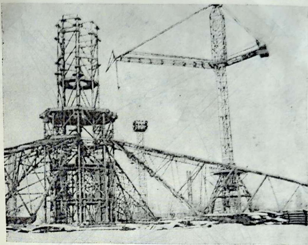
Рис. 70. Фрагмент смонтированной части башни.
