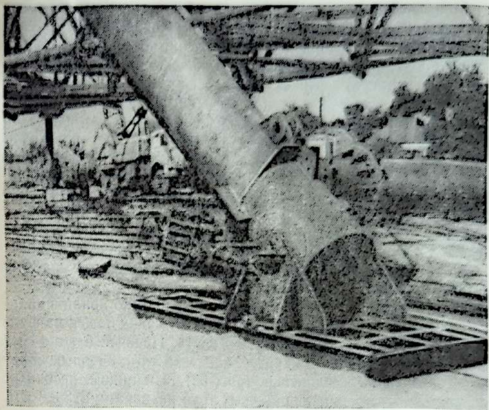
Рис. 65. Опорные салазки (общий вид).
