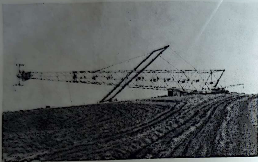
Рис. 64. Монтаж башни способом выжимания (общий вид).
