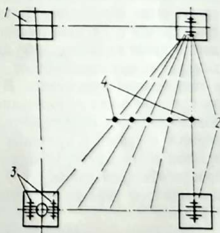
Рис. 67. Перераспределение нагрузки при включении в работу тормозного приспособления:
