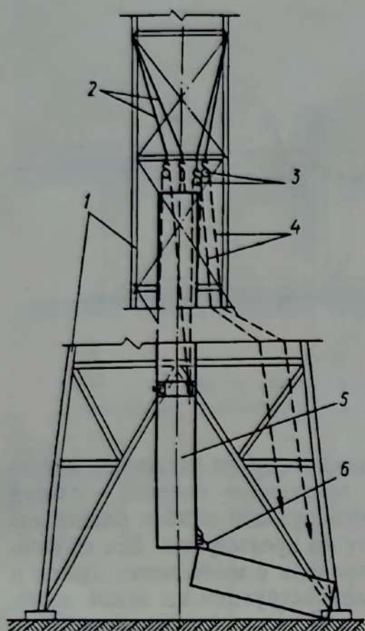
Рис. 79. Монтаж трубы газоотводящего ствола:
