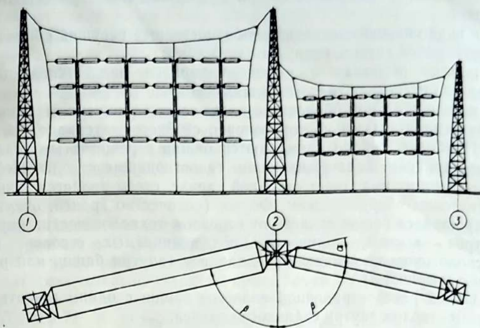
Рис. 4. Схема антенной цепочки антенн СГД 4/8 РА (подвеска антенных сетей выполнена на шарнирных траверсах).
