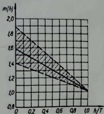
Рис. 24. Зависимость коэффициента m(h) приближенного учета динамического воздействия ветра от относительной высоты башни ( h отсчитывается от верха башни; T — высота башни).
