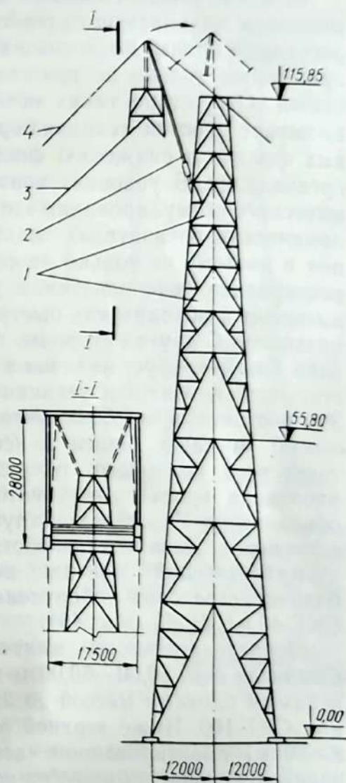
Рис. 48. Монтаж башни переставным порталом:
