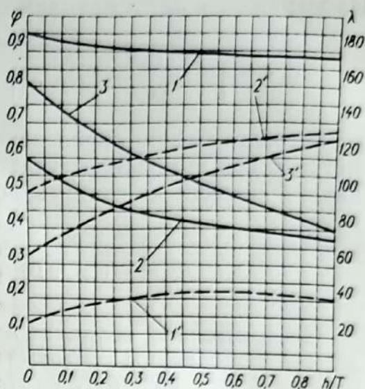
Рис. 26. Распределение усредненных значений гибкостей \lambda и коэффициентов продольного изгиба \varphi элементов башни по высоте ( h отсчитывается от верха башни):
