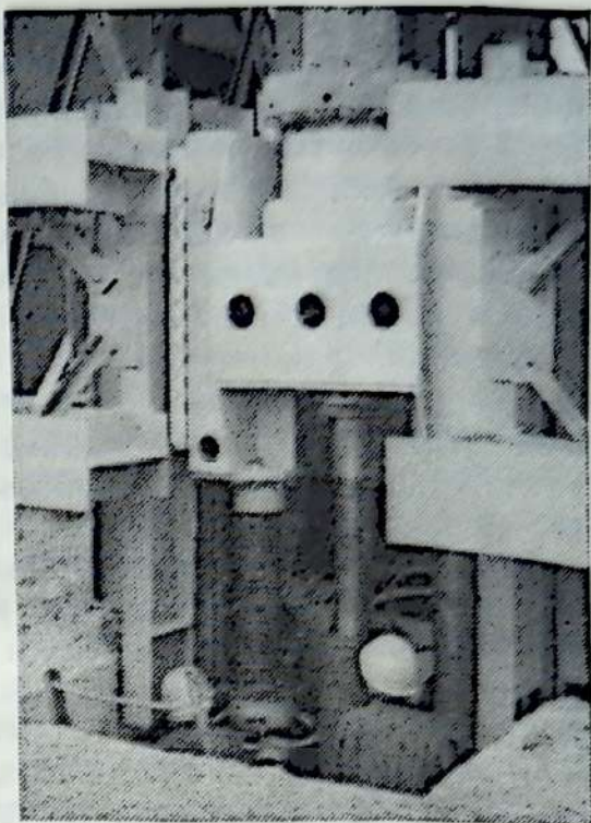
Рис. 74. Фрагмент гидродомкратной установки для подъема башни.
