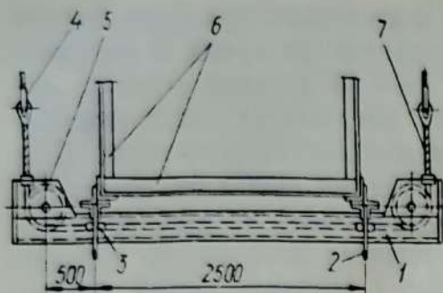
Рис. 35. Балансирная траверса: 1 — траверса из трубы; 2 — проушины; 3 — ограничители; 4 — крюк крана; 5 — ролики; 6 — конструкции башни; 7 — строп.
