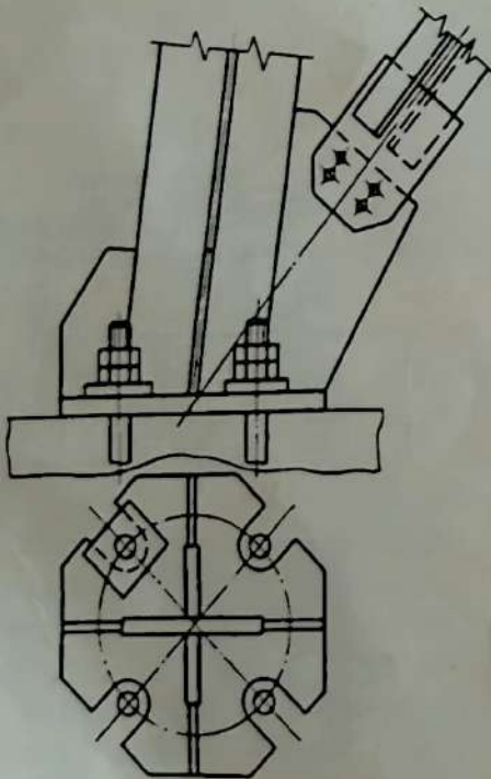
7. Опорный узел башни с поясами из электросварных сечений
