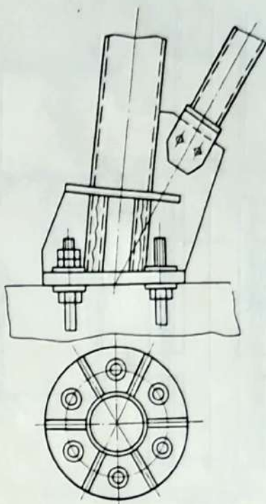
2. Опорный узел башни-трубы для химического производства
