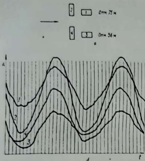
Рис. 22. Запись колебаний в ветровом потоке выхлопной башни-трубы высотой 150 м и диаметром газоотводящего ствола 2,6 м:
