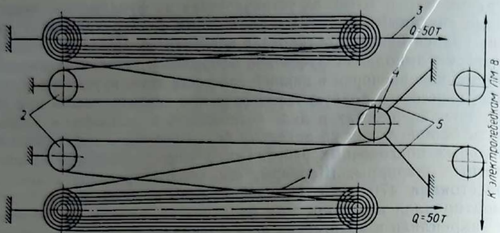
Рис. 61. Схема монтажных полиспастов П-1:
