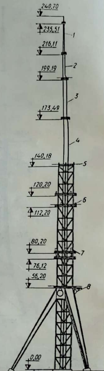
Рис. 15. Схема телевизионной башни в Харькове:
