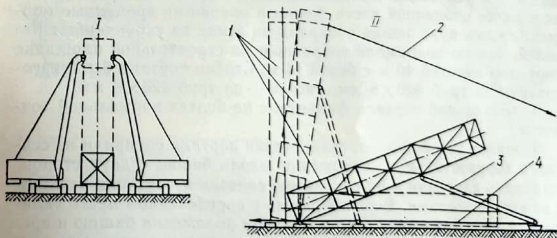
Рис. 62. Подъем башни способом выжимания с использованием толкателя: I — подъем башни кранами; II — выжимание башни толкателем; 1 — башня; 2 — тормозная оттяжка; 3 — толкатель; 4 — стягивающий полиспаст.
