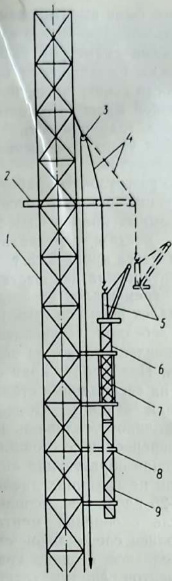
Рис. 43. Демонтаж ползучего крана:
