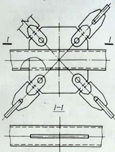
17. Узел пересечения с предварительно напряженными раскосами
