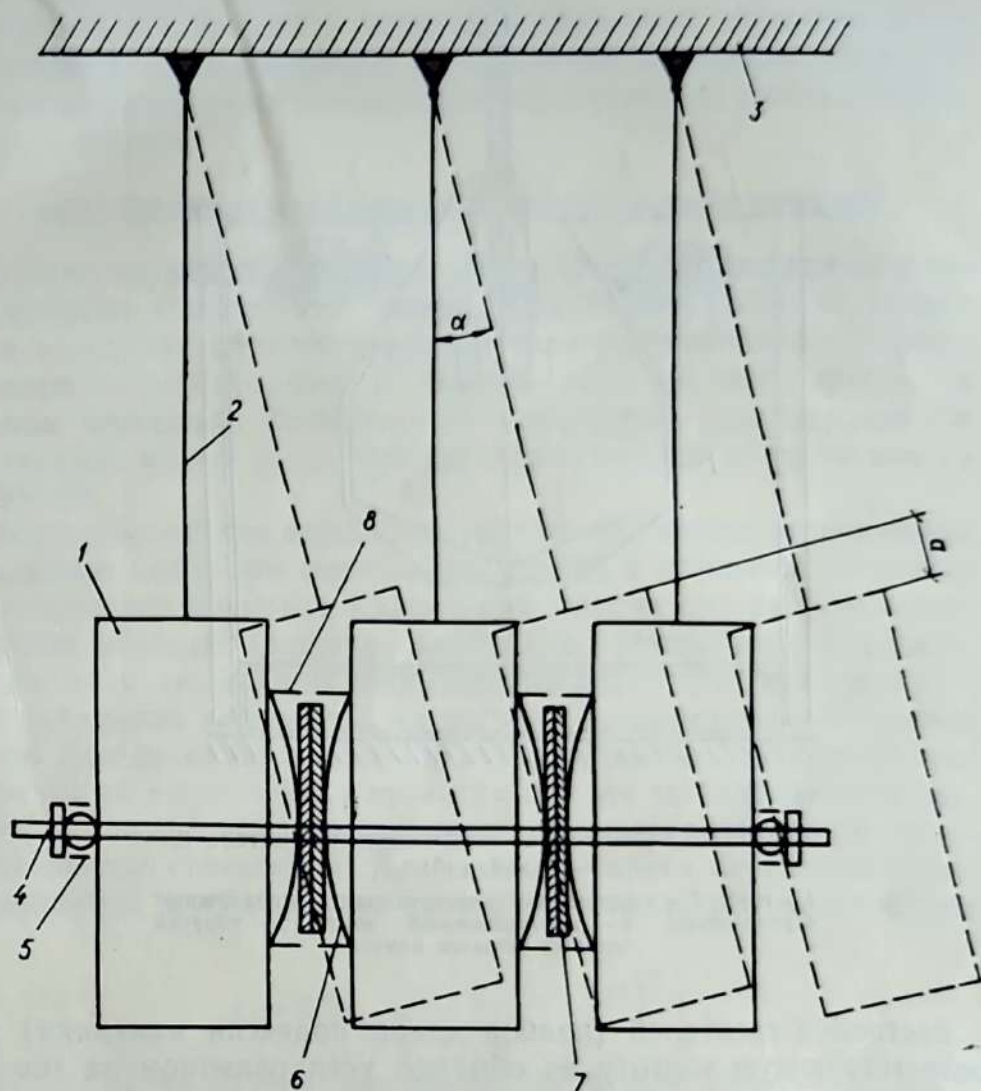
Рис. 20. Динамический гаситель колебаний маятникового типа: 1 — груз; 2 — подвеска; 3 — конструкция башни; 4 — винтовая стяжка; 5 — упор; 6 — пружины; 7 — фрикционные колодки; 8 — упоры для фиксации фрикционных колодок.
