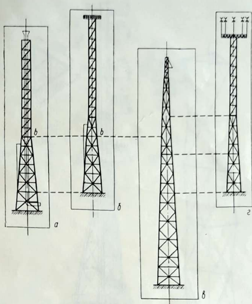
Рис. 10. Схемы башен, построенных на основе модульных схем: а — башня-труба; б — радиорелейная опора; в — башня для антенн СГД; г — башня для антенн «Алтай».
