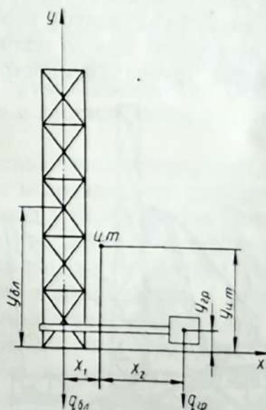
Рис. 33. Определение координат центра тяжести системы (блок + дополнительный груз).
