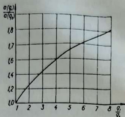
Рис. 28. Зависимость относительного поперечного размера башни a от изменения нагрузки q .
