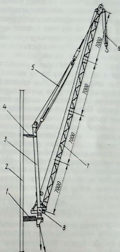
Рис. 41. Переставной стреловой кран: 1 — нижний опорный столик; 2 — пояс башни; 3 — стойка крана; 4 — верхний столик; 5 — стреловой полиспаст; 6 — грузовой полиспаст; 7 — стрела; 8 — поворотный круг.
