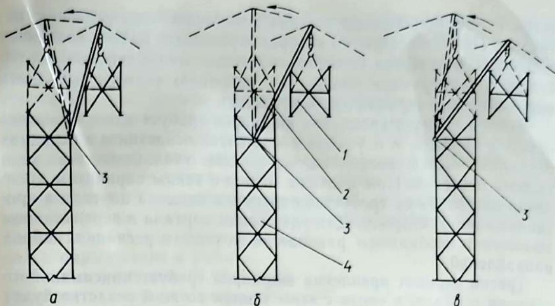
Рис. 47. Схемы крепления портала (а—в — варианты):
