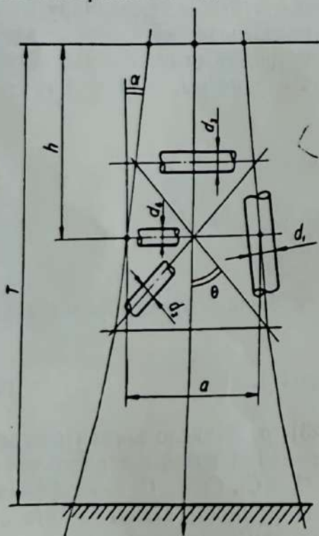
Рис. 23. Расчетная модель для формирования нагрузок и определения усилий при оптимизации.
