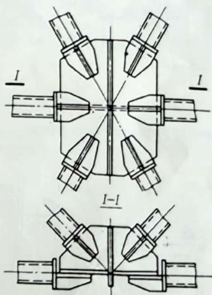
20. Узел пересечения раскосов с промежуточными распорками со сварной вставкой из стальных листов [6]
