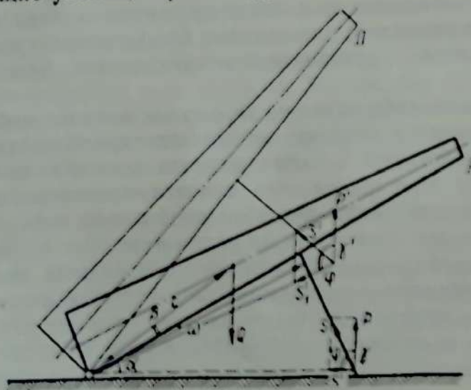
Рис. 38. Расчетная схема усилий при монтаже башни поворотом вокруг шарниров через рамную подставку с дотягиванием полиспастом.
