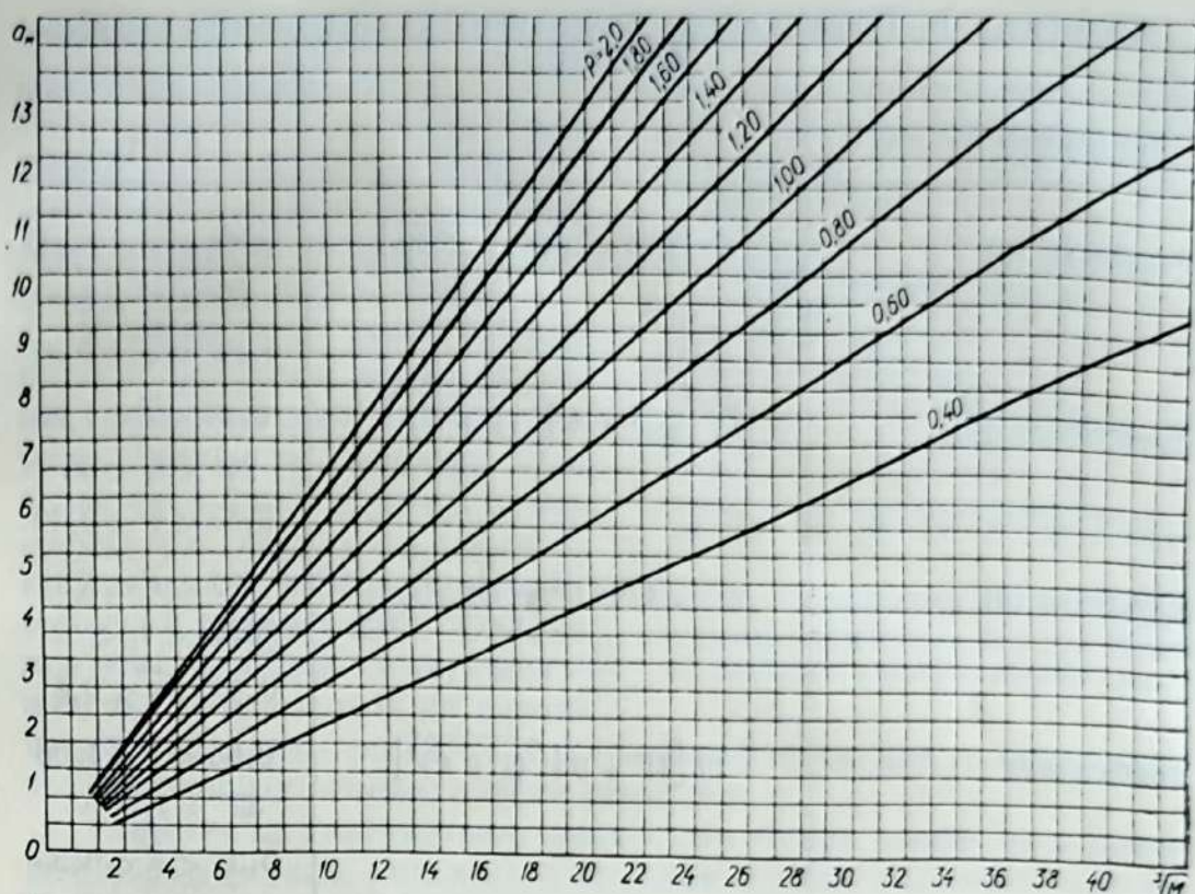
Рис. 29. Зависимость поперечного размера башни a от изгибающего момента M , вычисленного в направлении «на грань» (при k=0,4 \cdot 10^{-4} ; R=2,1 \cdot 10^4 тс/м 2 ; \varphi(t)=0,40 — для треугольной решетки).
