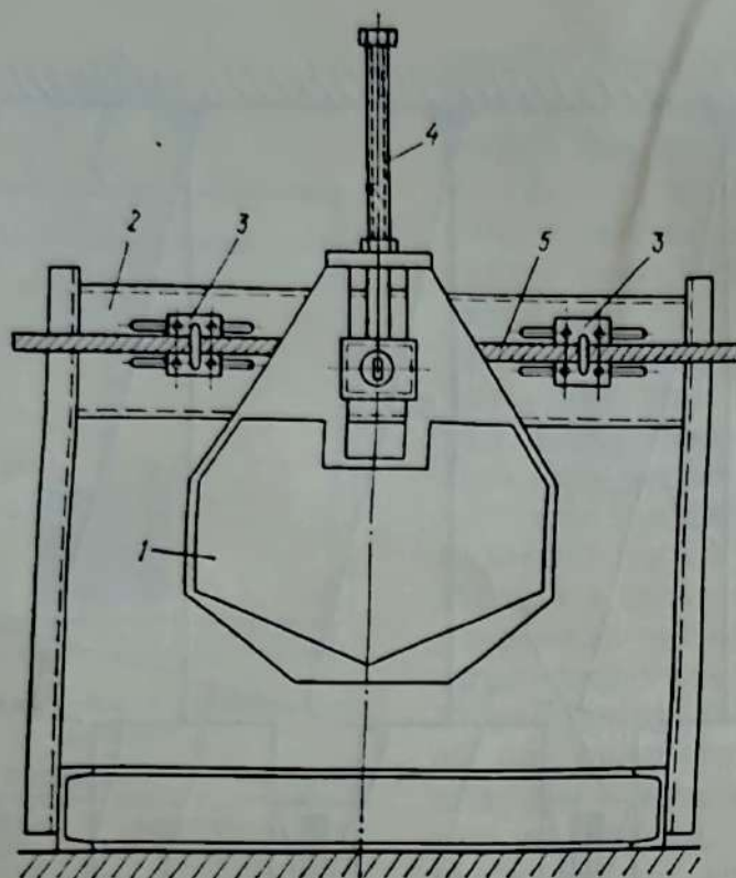
Рис. 21. Динамический маятниковый гаситель колебаний:
