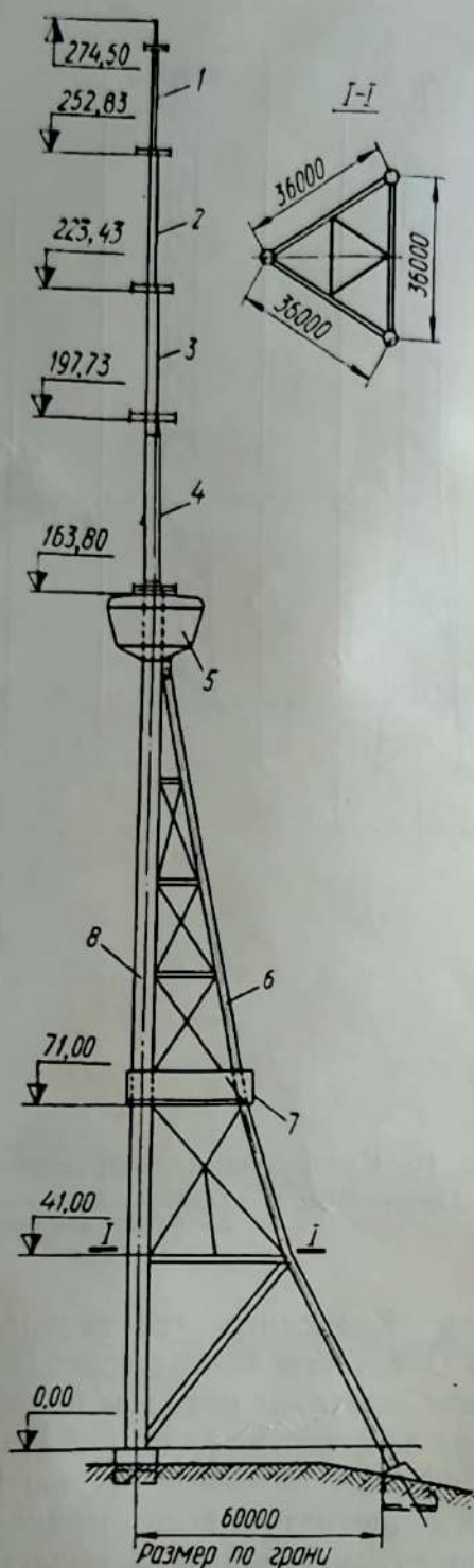
Рис. 12. Схема телевизионной башни в Тбилиси:
