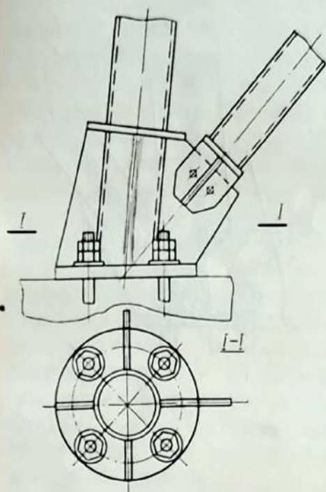
3. Опорный узел башни-трубы с траверсами для анкерных болтов [6]
