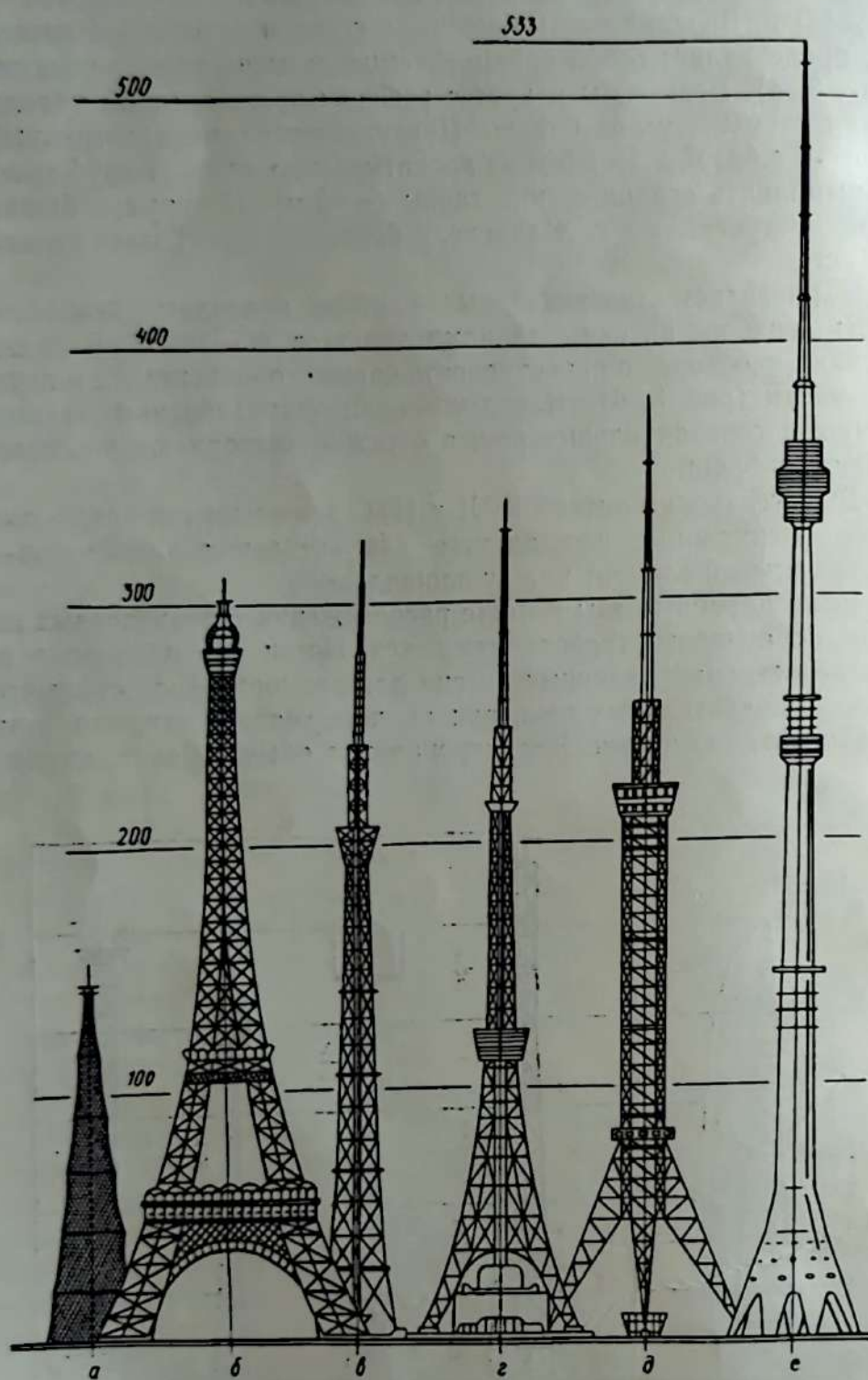
Рис. 2. Уникальные радиотелевизионные башни (высота дана в м): а — радиобашня Шухова в Москве; б — Эйфелева башня в Париже; в — телевизионная башня в Ленинграде; г — телевизионная башня в Токио; д — телевизионная башня в Киеве; е — телевизионная башня в Останкино (Москва).
