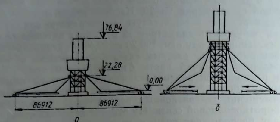
Рис. 68. Монтаж башни способом подращивания:
