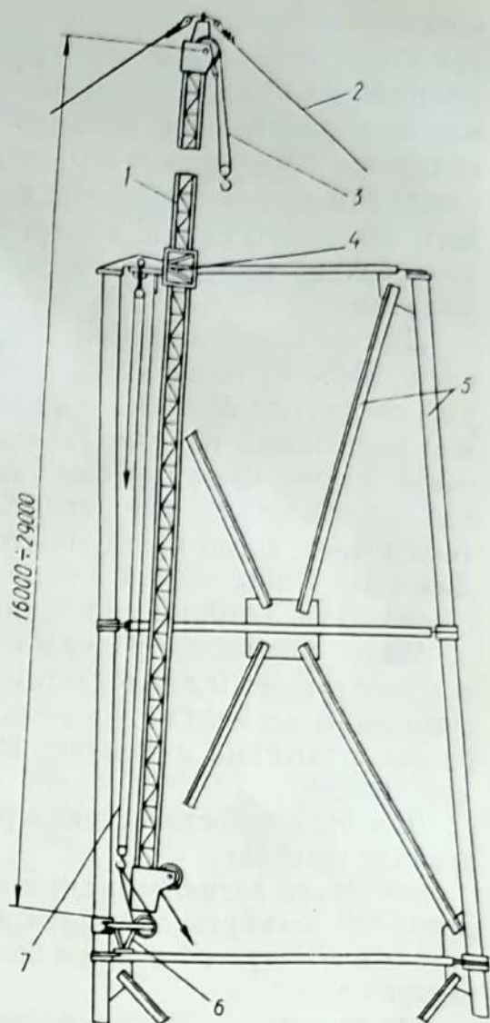
Рис. 40. Закрепление монтажной мачты:
