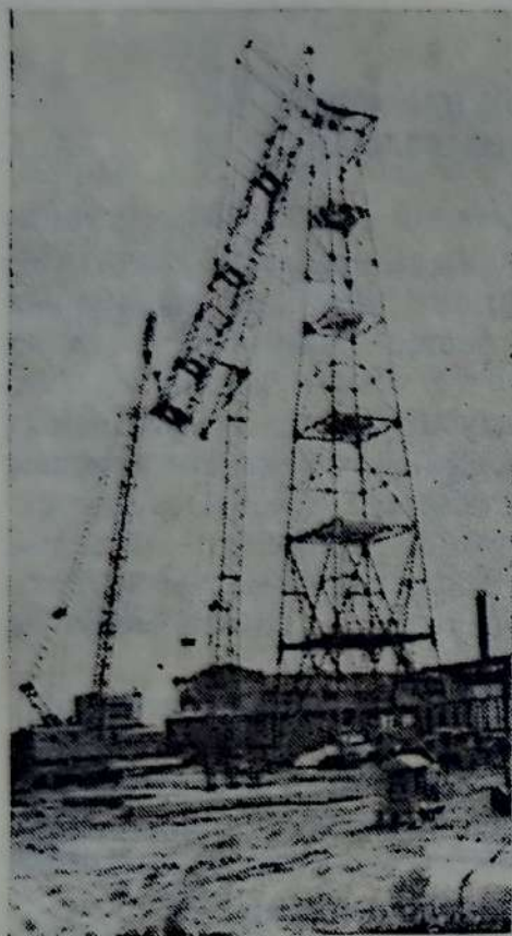
Рис. 80. Установка верхнего блока башни в шарниры.
