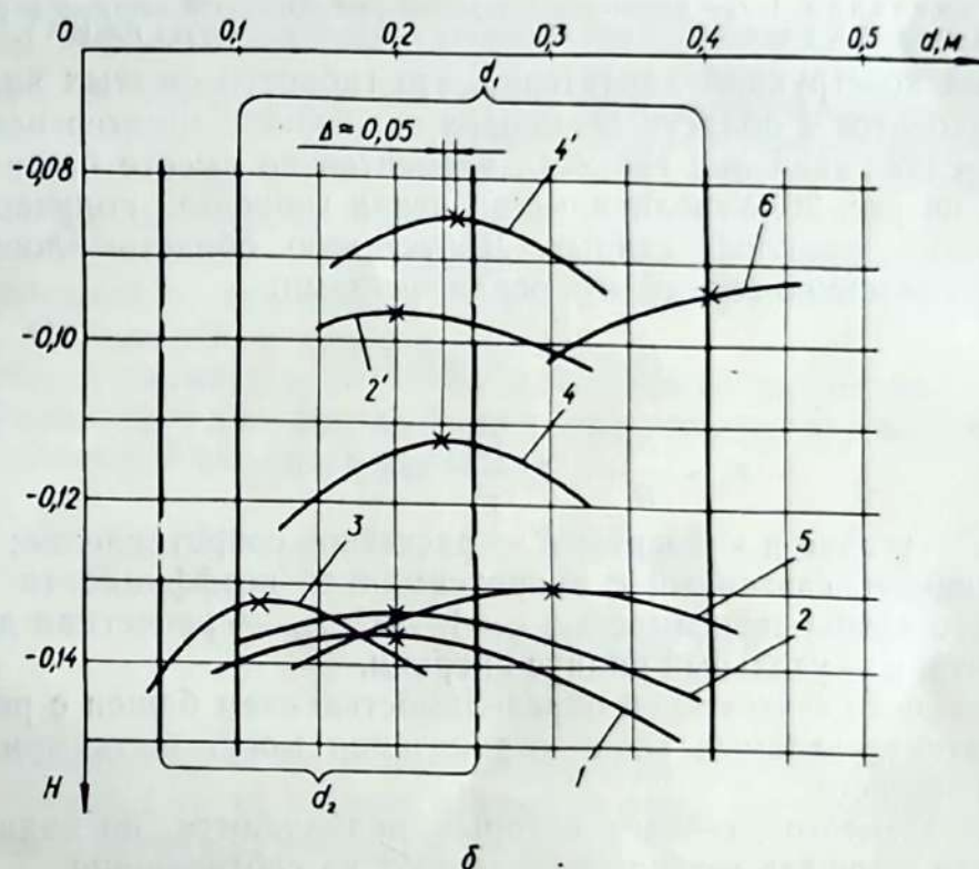
Рис. 25. Сопряженные функции и функции Гамильтона:
