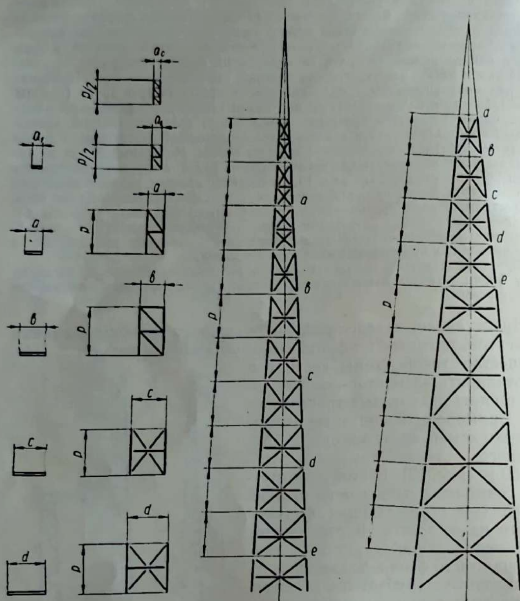
Рис. 9. Модульные схемы для построения башен (буквами обозначены поперечные размеры панелей).
