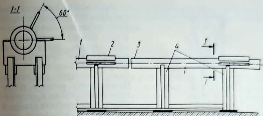
Рис. 78. Кондуктор для сборки элементов поясов: 1 — пояс башни; 2 — узловая фасонка; 3 — стык поясов; 4 — кондуктор.
