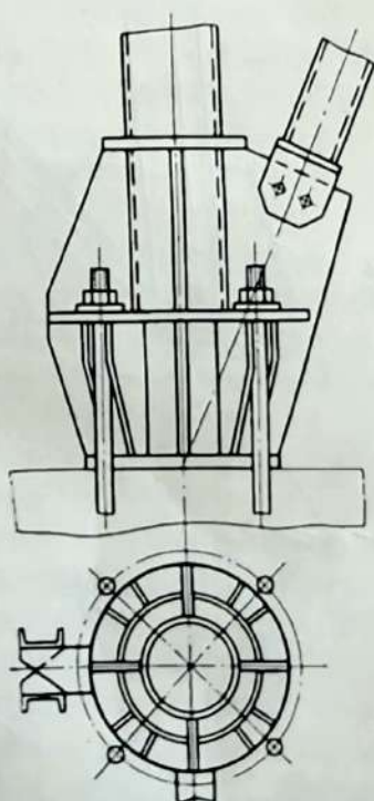
3. Опорный узел башни-трубы с траверсами для анкерных болтов [6]
